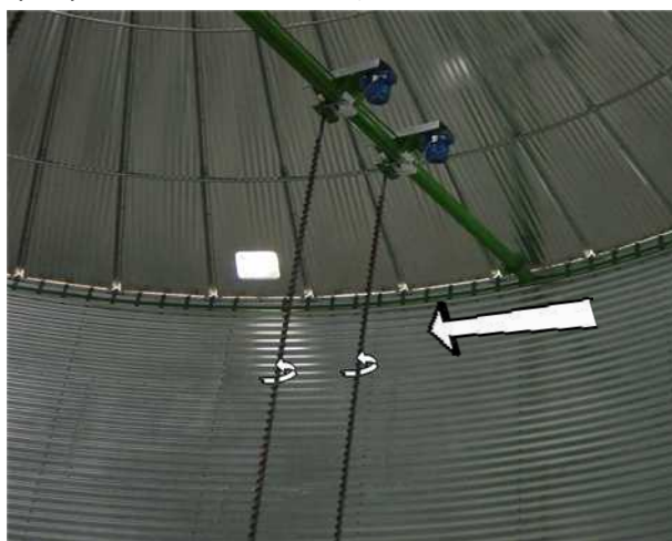
(DK) Omrøresystem med omrøresnegle (UK) Stirring system w. down augers (DE) Rührsystem mit Rührschnece
